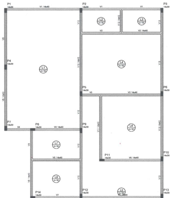
Forma do pavimento 1º Andar (Nível 290)
