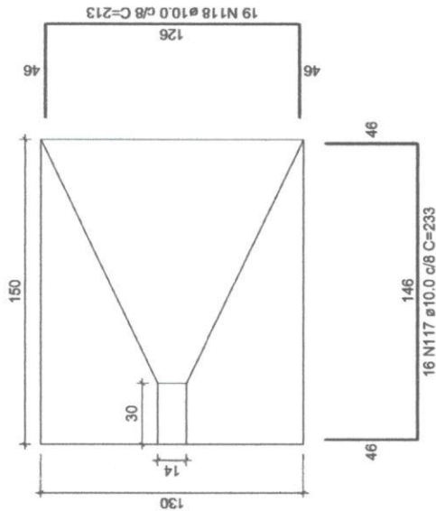
S12 PLANTA ESC 1:25
