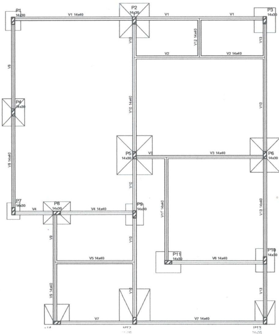
Forma do pavimento Baldrame
